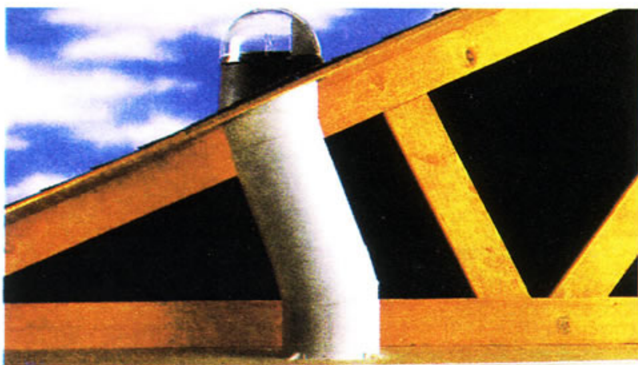
La longitud de construcción máxima recomendada del Solatube 10" es de 2,5 m.
